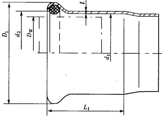
图 B.0.1 不锈钢卡压式管件承口
