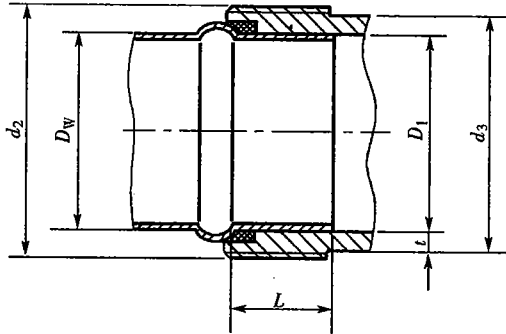
图 C.0.1 不锈钢压缩式管件承口
